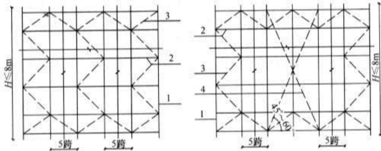
图 6.1.3-1 满堂架高度不大于 8m 斜杆设置立面图 图 6.1.3-2 满堂架高度不大于 8m 剪刀撑设置立面图
