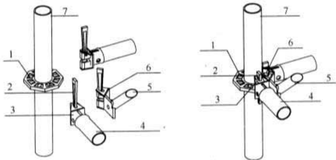
图 3.1.1 盘扣节点
