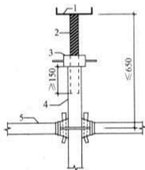
图 6.1.5 带可调托座伸出顶层水平杆的悬臂长度 1—可调托座；2—螺栓；3—调节螺母；4—立杆；5—水平杆
