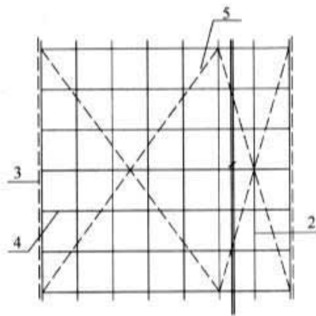
图 6.2.3-2 每 5 跨设扣 件钢管剪刀撑
