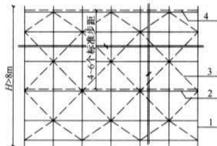
图 6.1.3-3 满堂架高度大于 8m 水平斜杆设置立面图 1—立杆；2—水平杆；3—斜杆；4—水平层斜杆或扣件钢管剪刀撑
