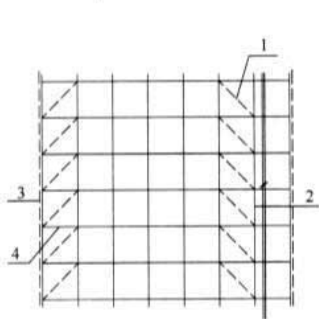
图 6.2.3-1 每 5 跨 每层设斜杆
