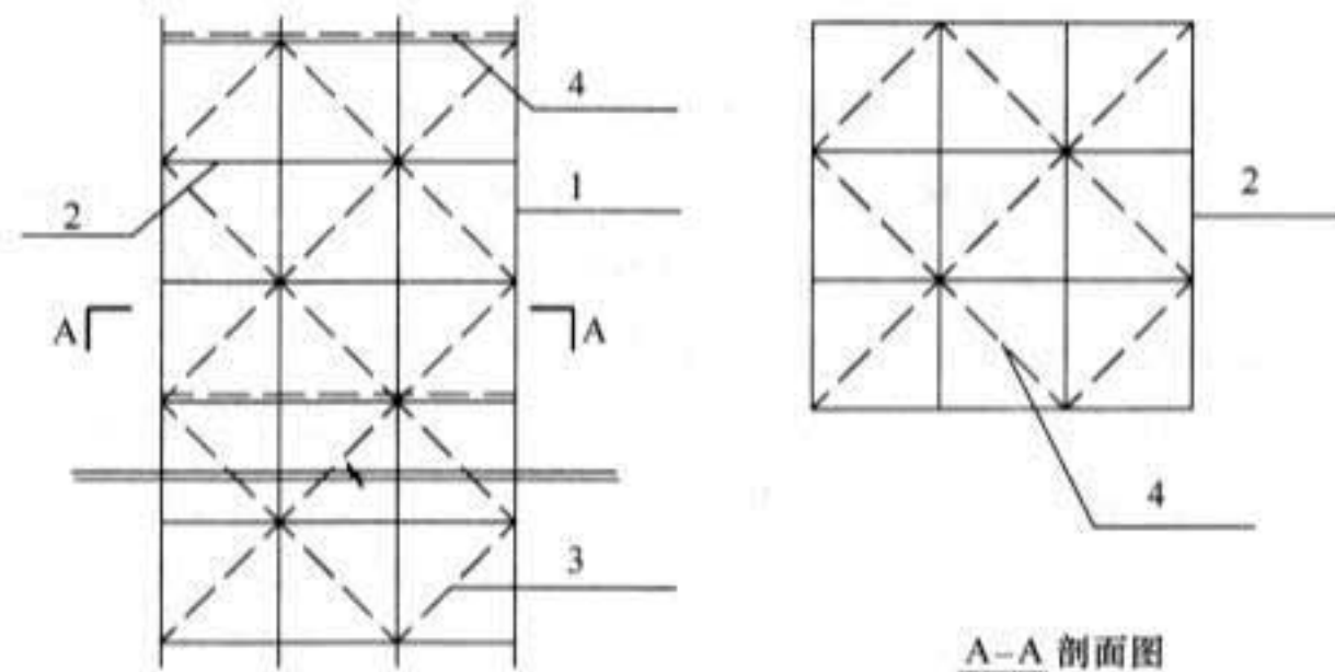
图 6.1.3-4 无侧向拉结塔状支模架 1—立杆；2—水平杆；3—斜杆；4—水平层斜杆
